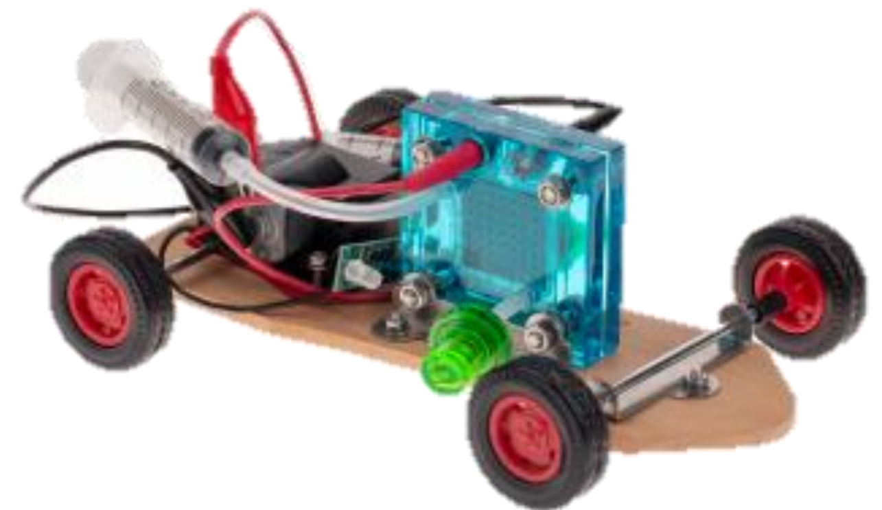
První prototyp vašeho vodíkového autíčka
